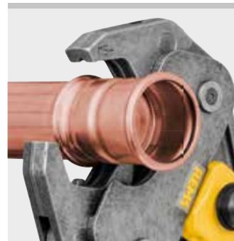
Пресс-клещи REMS (4G)
